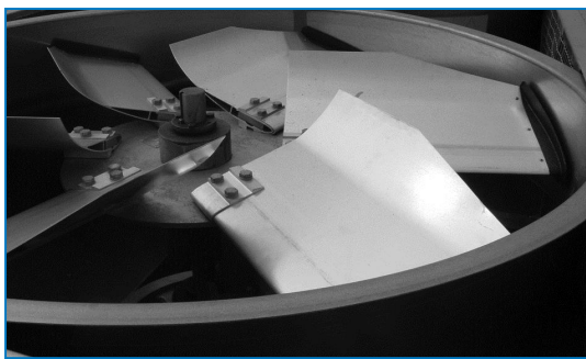
Axial Fan
